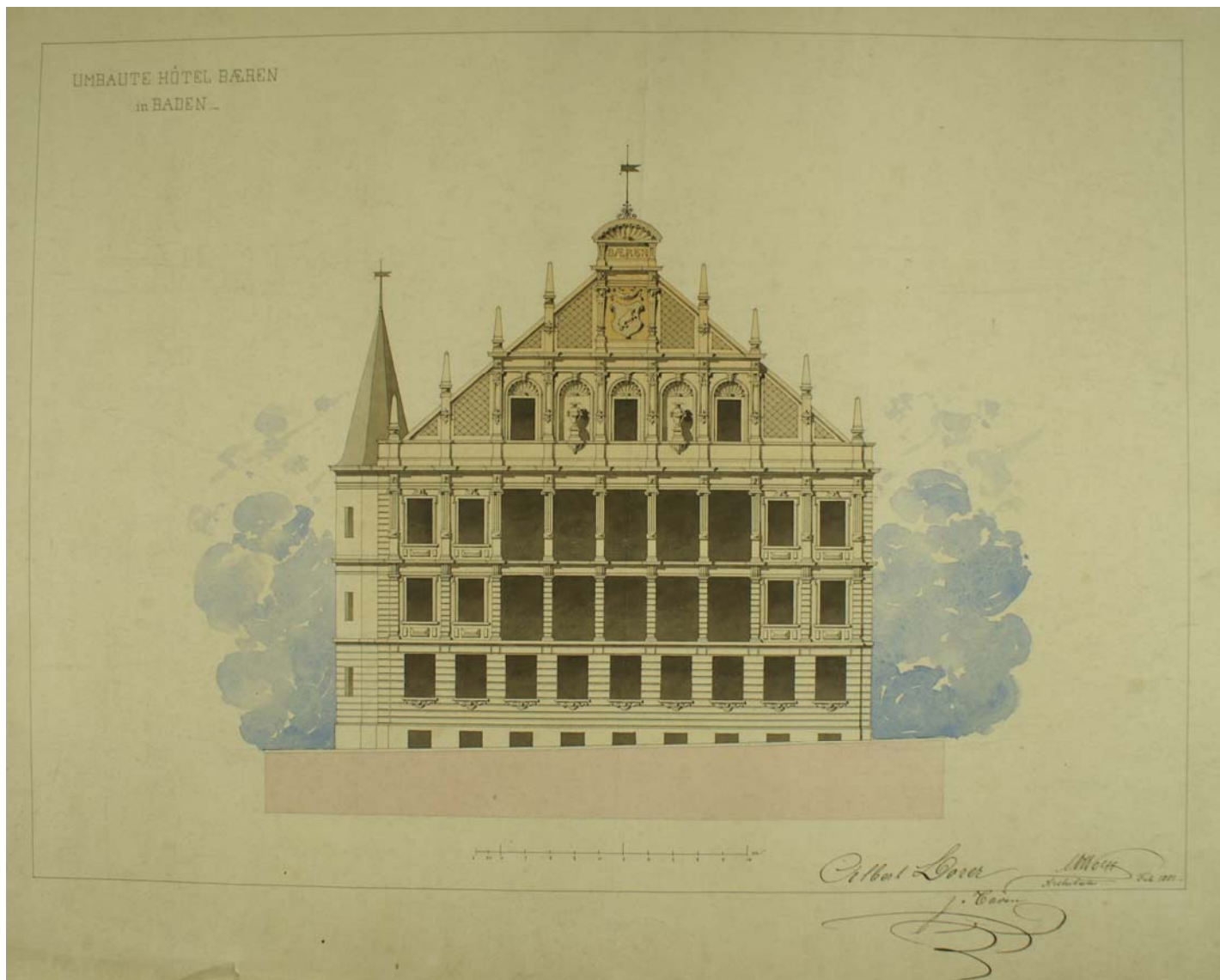
Zeichnung der Neorenaissancefassade des „Bären“; Baueingabe durch den Architekten Wolff. Original Stadtarchiv Baden.
